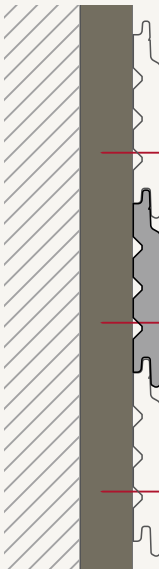
Largeur utile ≤ 125 mm et épaisseur ≤ 28 mm Sans finition
